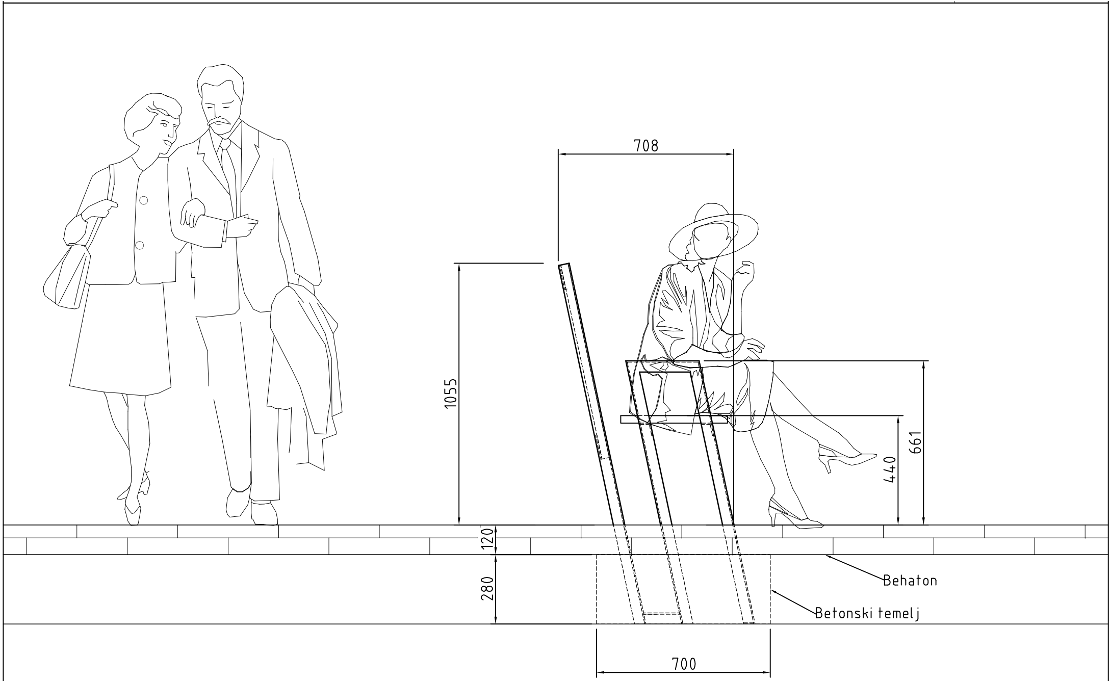
Varijanta klupe sa betoniranjem dela konstrukcije
