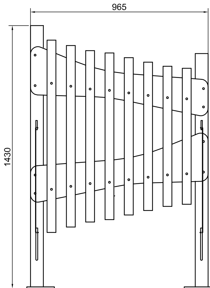
Frontalni pogled
