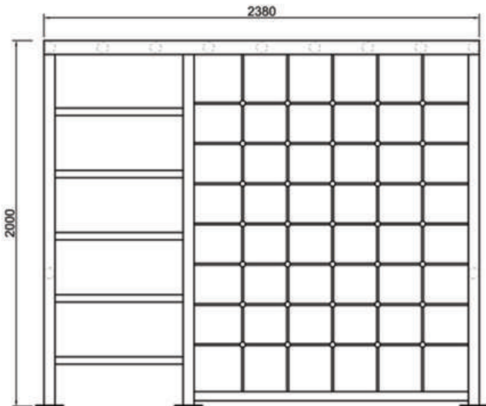
penjalica - pogled
