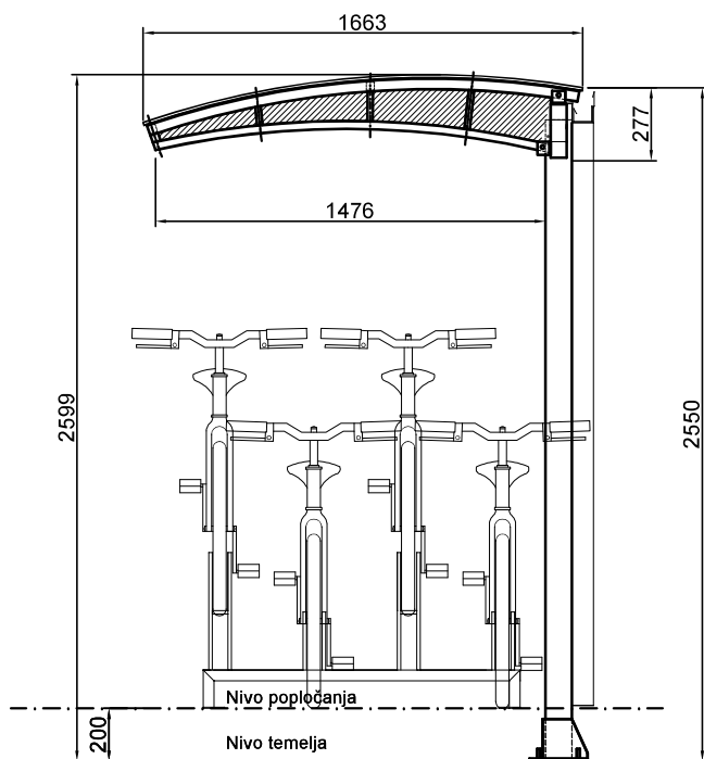
Bočni pogled
