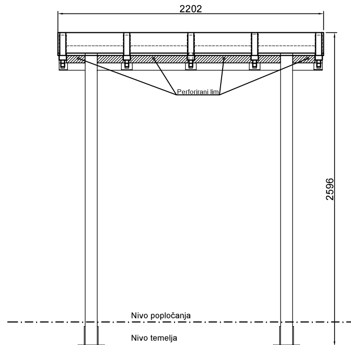
Frontalni pogled
