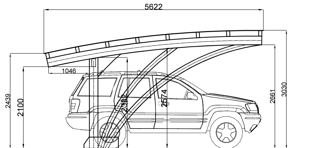
Bočni pogled - Varijanta sa lučnim nosačima
