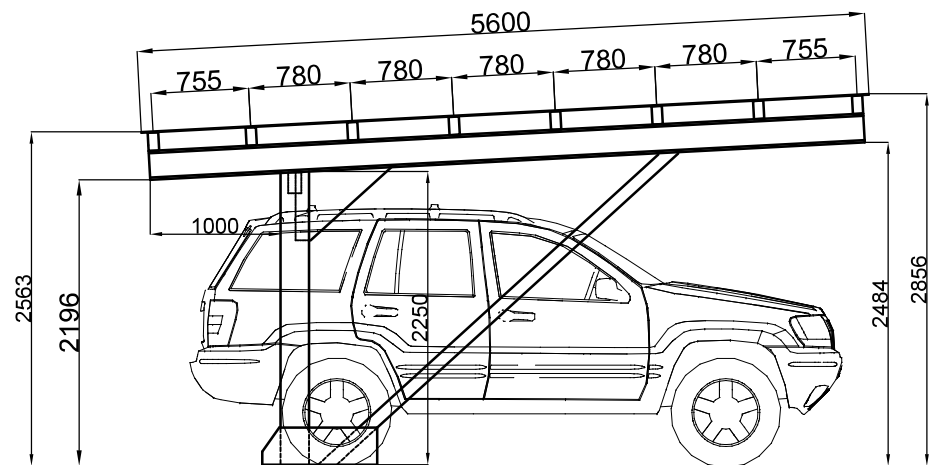
Bočni pogled-Varijanta sa ravnim nosačima
