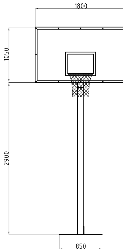
FRONTALNI POGLED
