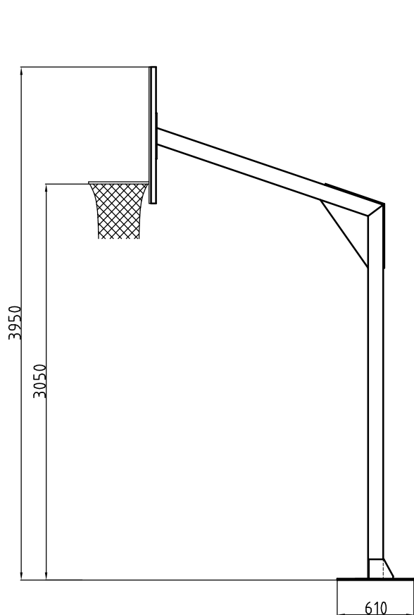
BOČNI POGLED
